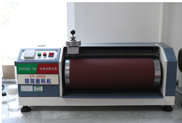
辊筒磨耗机 Roller abrasion machine
